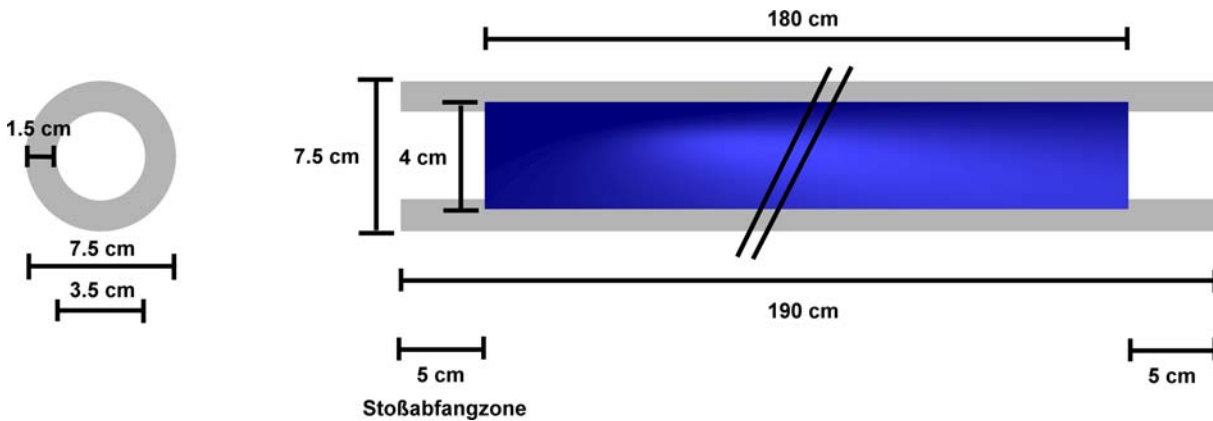
Skizze zum Bau eines Safty-Bo's.
